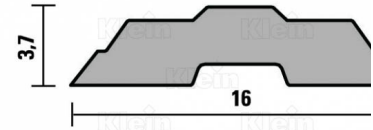
TURNBLADES "VARIPLAN"
